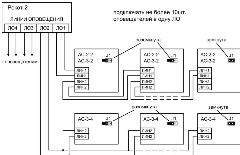
Рис.А3 Схема подключения оповещателей «АС-2-2», «АС-3-2», «АС-3-4» (параллельное соединение)
