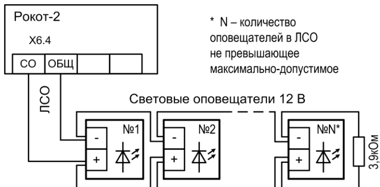
Рис.А5 Схема подключения световых оповещателей к ЛСО
