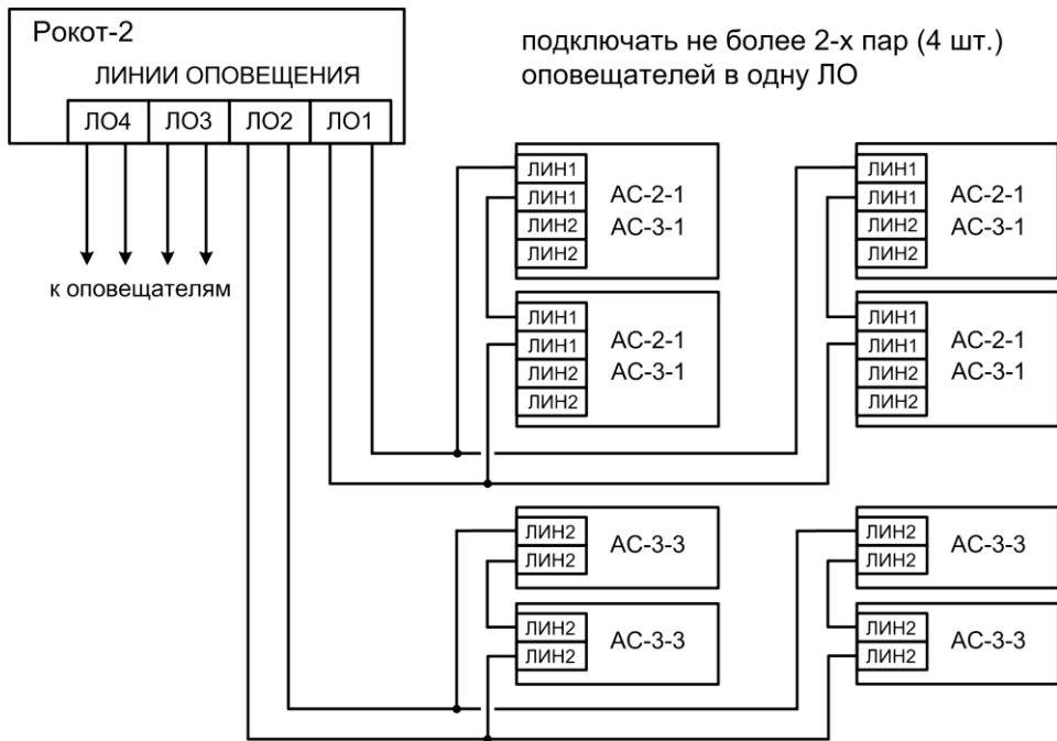
Рис.А4 Схема подключения оповещателей «АС-2-1», «АС-3-1», «АС-3-3» (параллельно-последовательное соединение)
